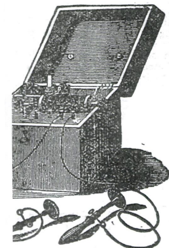
Induktionsapparat med element i lädan. Pris kr. pr st. 125.
